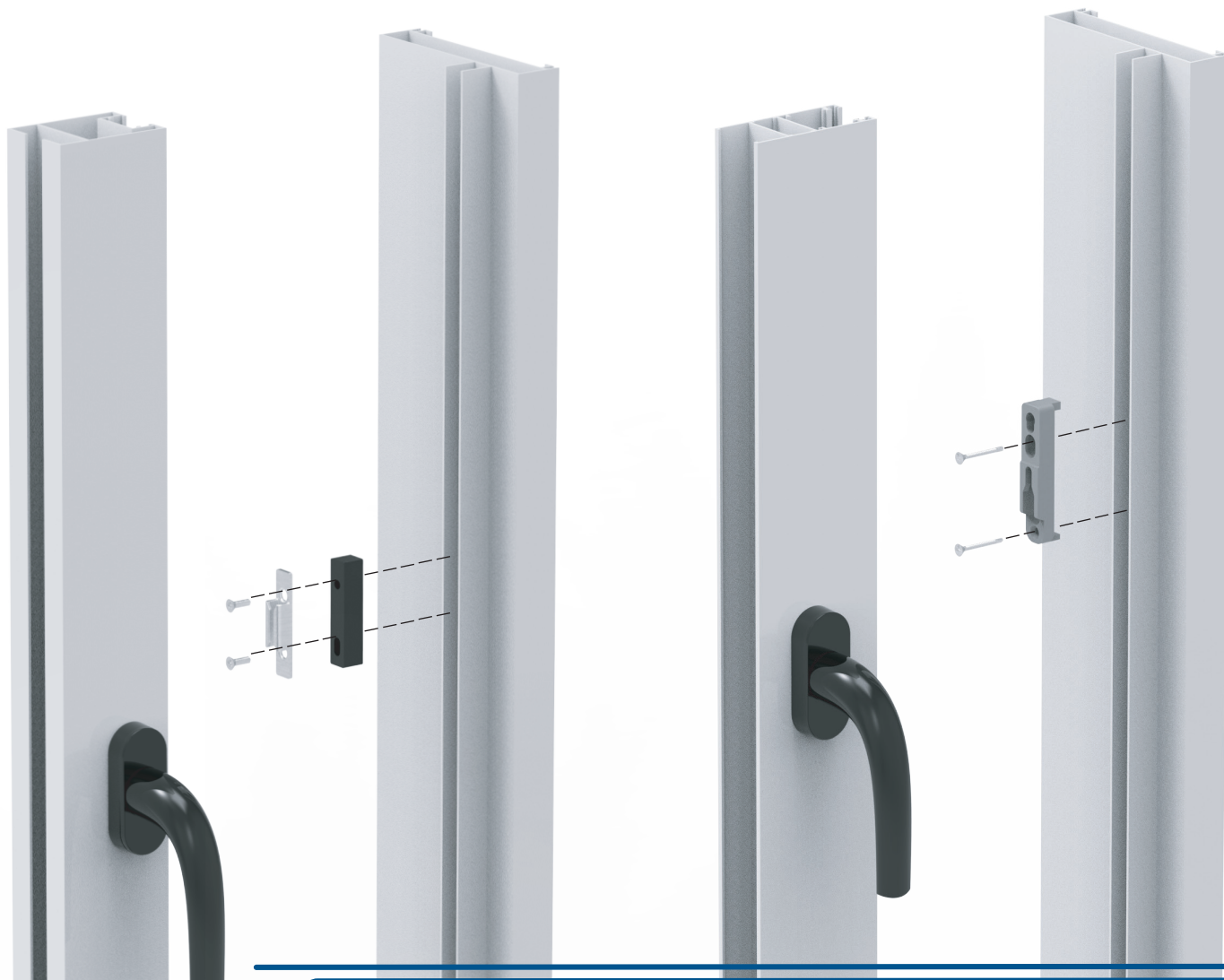
CERRADERO PERIMETRAL + SUPLEMENTO A40 90°
