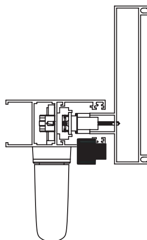
CERRADERO PLÁSTICO HA62 45°- MARCO 90°
