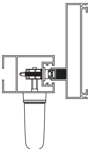
CERRADERO PERIMETRAL + SUPLEMENTO A40 90°
