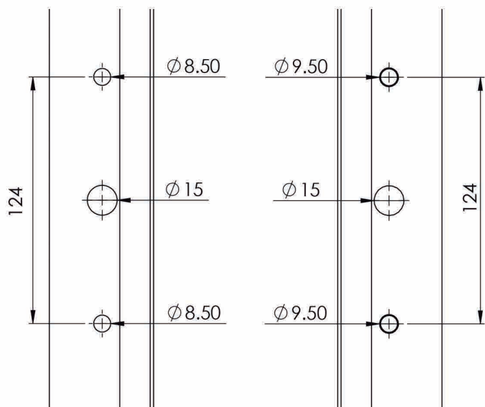
MEDIDAS MECANIZADO PARA MANIJA EN MODENA 90°
