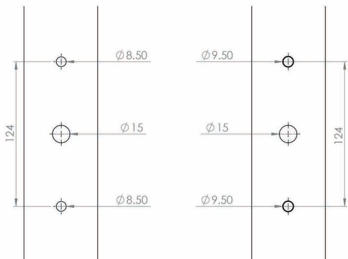
MEDIDAS MECANIZADO PARA MANIJA EN A-40 / HA-62
