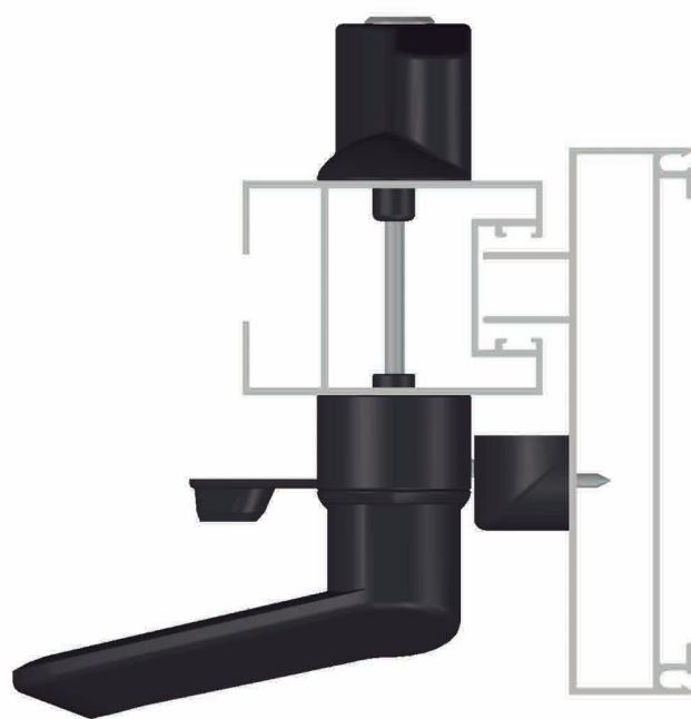
VISTA SUPERIOR CONJUNTO
