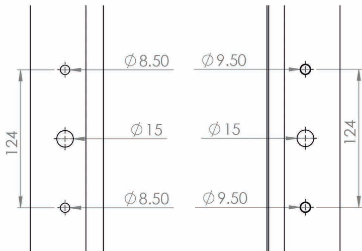
MEDIDAS MECANZADO PARA MANIJA EN A-30
