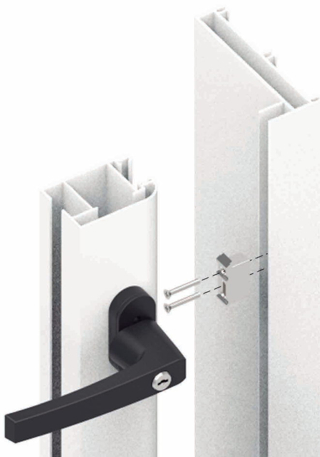
MEDIDAS CERRADERO
