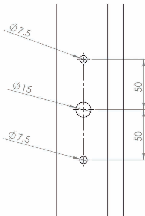
MEDIDAS CALADO EN A-30NEW
