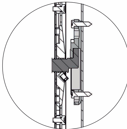
CORTE DETALLE GANCHO DE CIERRE CON CERRADERO
