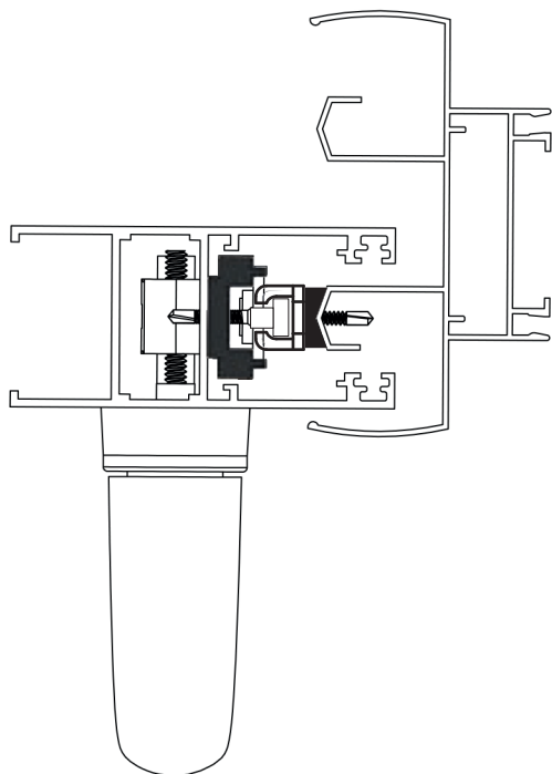
VISTA SUPERIOR CONJUNTO
