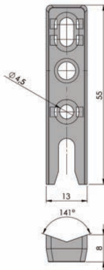
MEDIDAS CERRADERO
