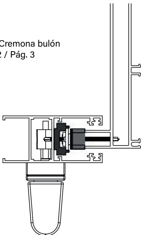
VISTA SUPERIOR CONJUNTO
