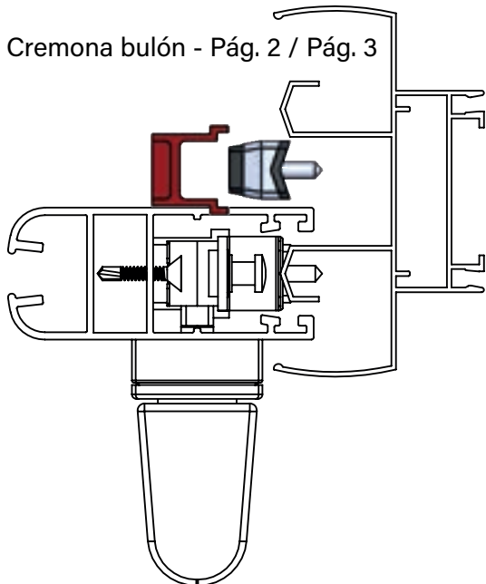
VISTA SUPERIOR CONJUNTO
