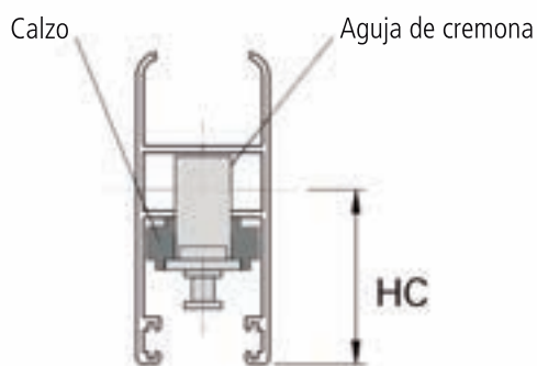
CONJUNTO
