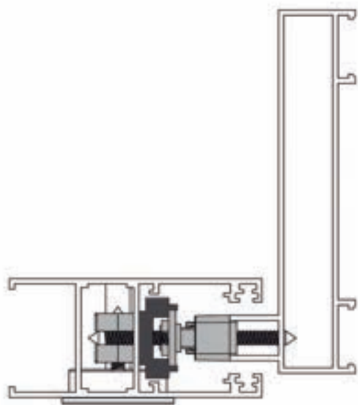
VISTA SUPERIOR CONJUNTO
