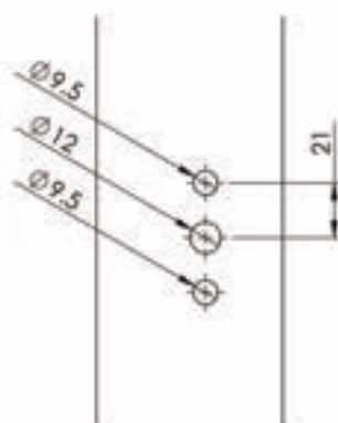
MEDIDAS CALADO EN JAMBA 45°
