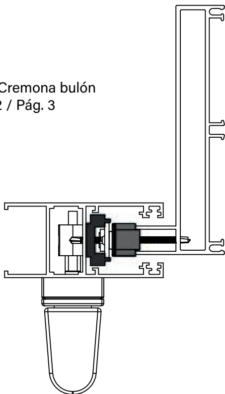
VISTA SUPERIOR CONJUNTO
