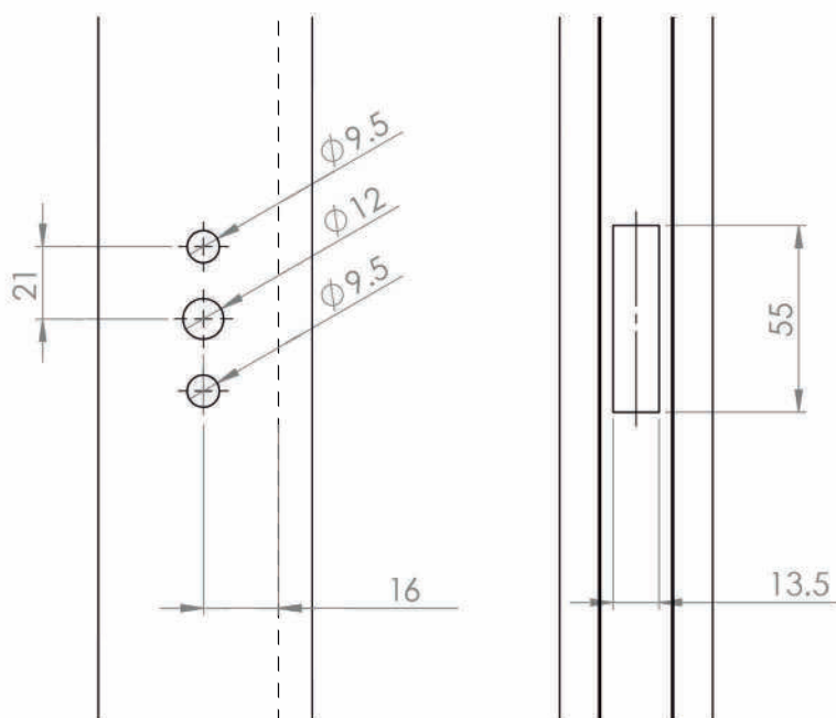
MEDIDAS MECANIZADO
