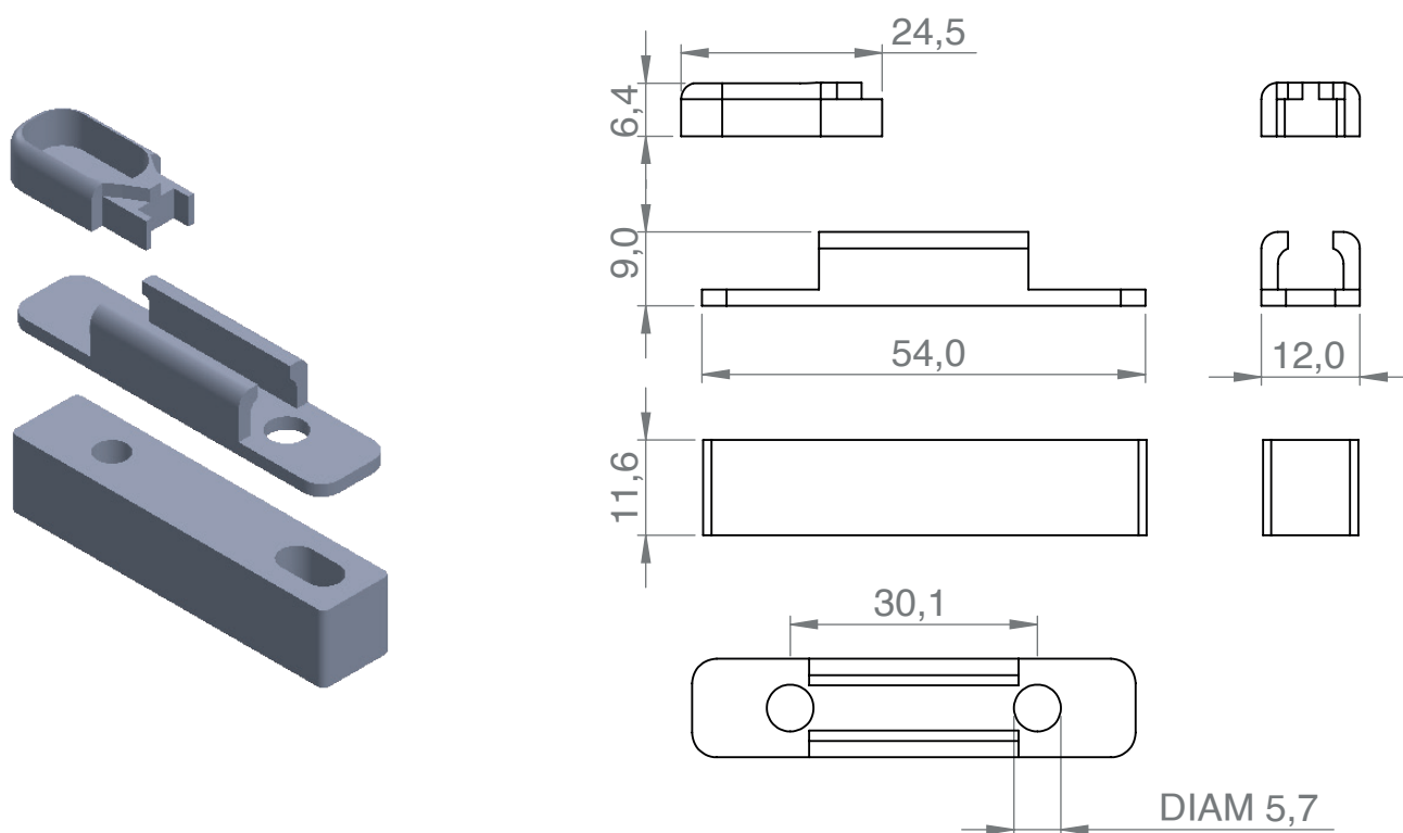
Cerradero Aluminio Zamak y Plástico - PERIMETRAL - COD CGK002
