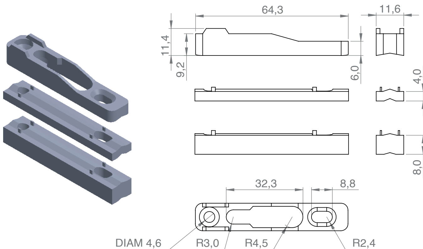
Cerradero Aluminio Zamak y Plástico - UNIVERSAL - COD 13230142
