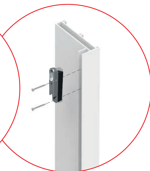
Cerradero Aluminio Zamak y Plástico - PERIMETRAL COD CGK002
